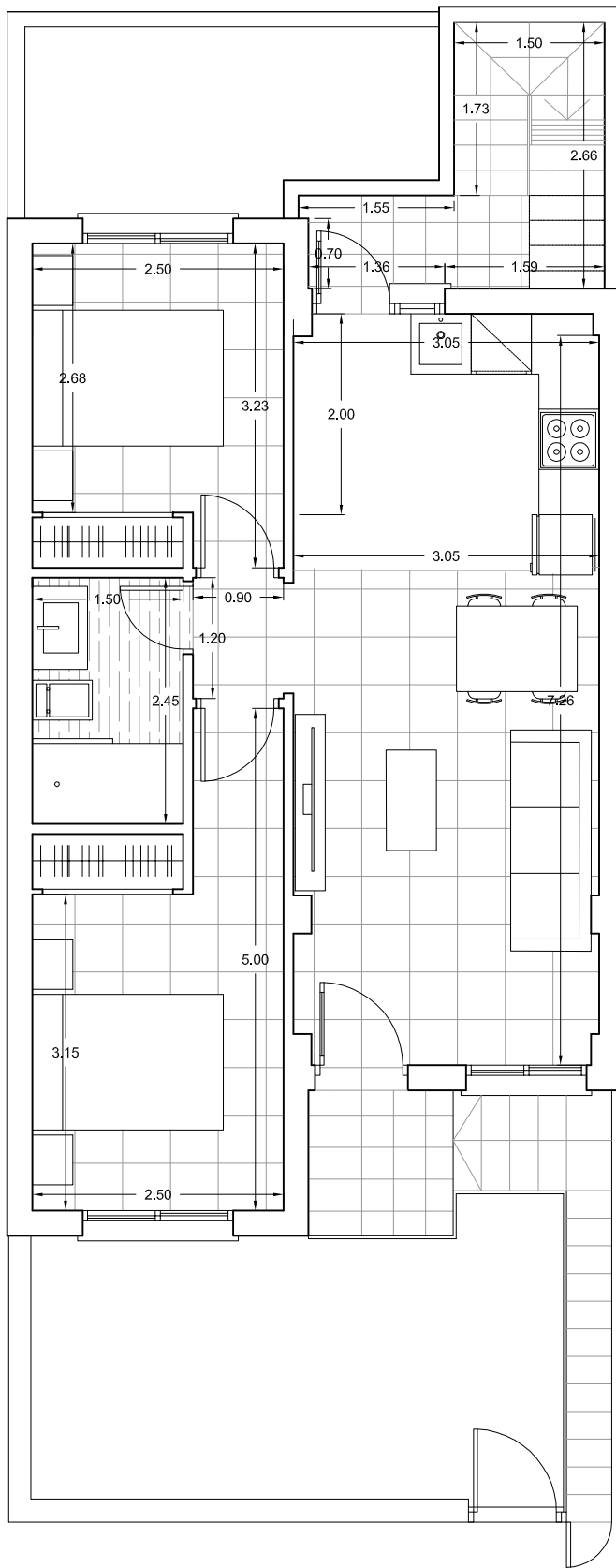
VIVIENDA 5 PP
