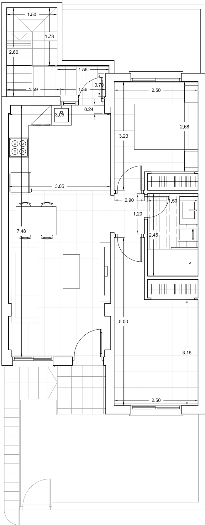
VIVIENDA 2 PP
